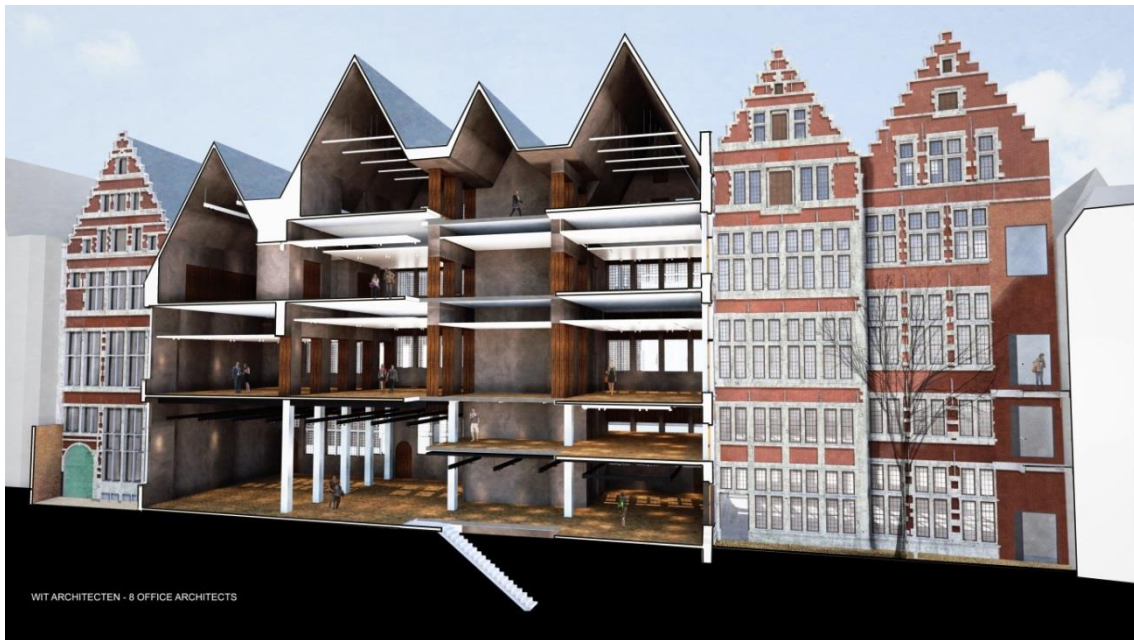
Coupe des salles d'exposition DIVA © DIVA / TV WIT architecten – 8 office architects Rez-de-chaussée & 1 er étage salles d'exposition collection permanente A Brilliant Story 2 e & 3 e étages salles d'expositions temporaires 4 e étage laboratoire de conservation et restauration
